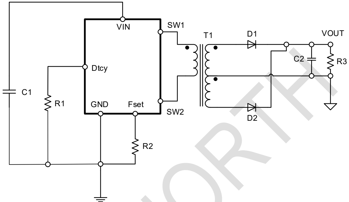
图 12-1 应用原理图
