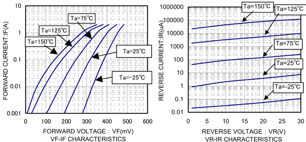
图 12-2 肖特基 RB060M-30 工作特性曲线
