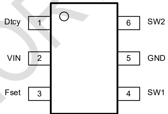
SOT23-6
