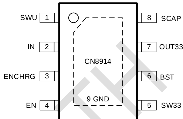
图 1 ESOP8L
