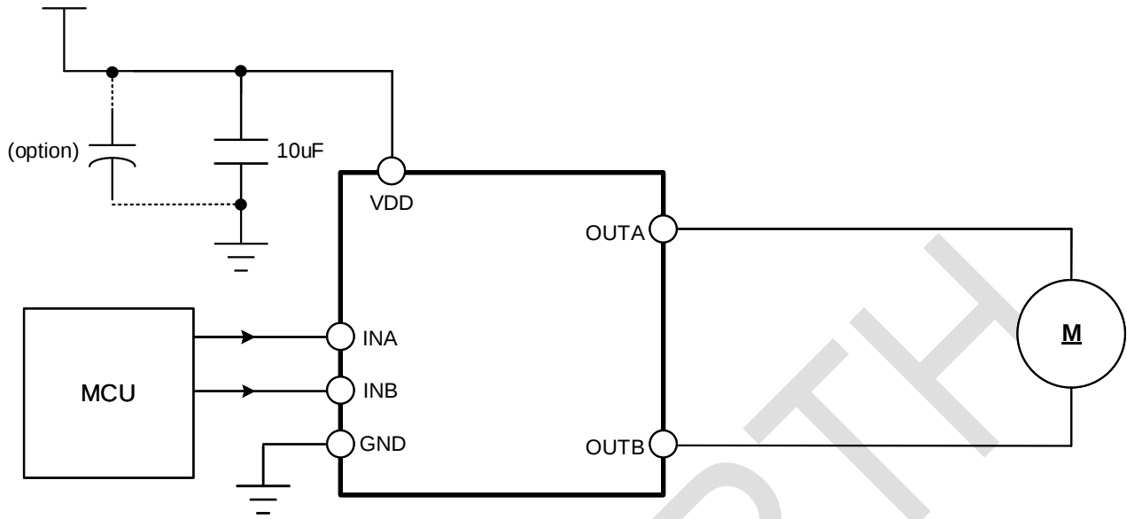
典型应用图
